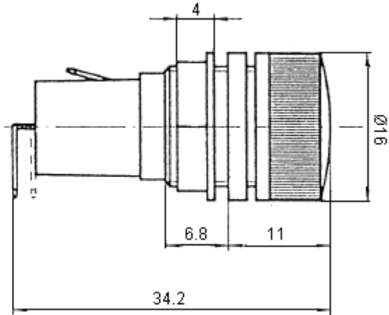
Dimensions : Millimetres
