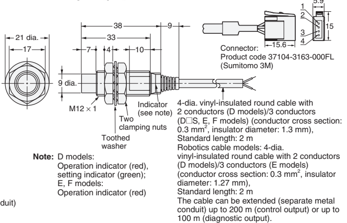
Fig. 9 : E2E-X8MD□ E2E-X5ME□/F□
