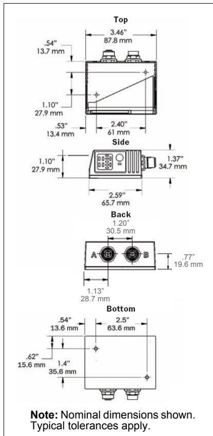
QX-830 Dimensions
