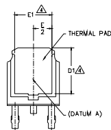
VIEW A-A
