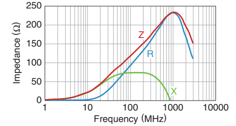
MMZ0603S601C
