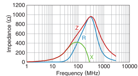
MMZ1005Y601C
