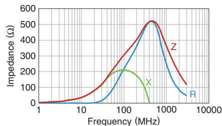
MMZ1005Y301C
