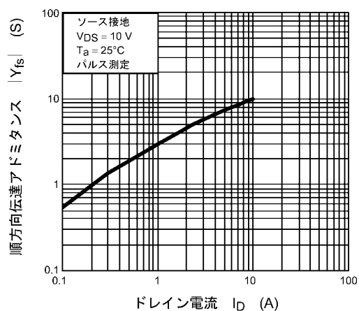
図 8.5 |Y_{fs}| - I_D
