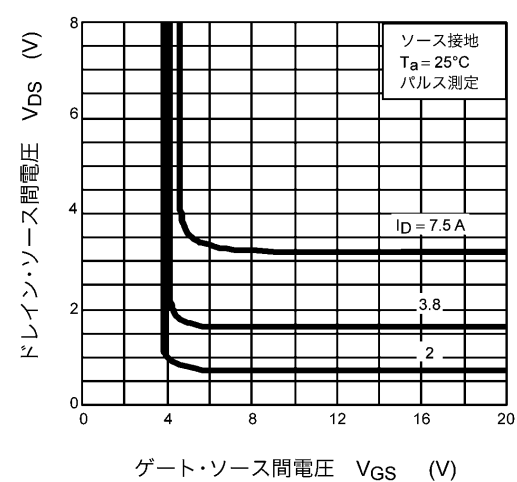
図 8.4 V_{DS} - V_{GS}
