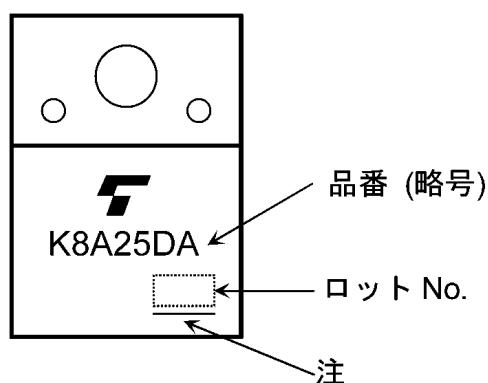
図 7.1 現品表示
