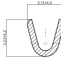
SECTION A-A 4:1
