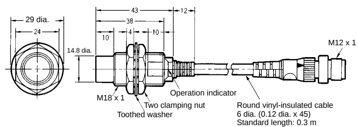
Fig. 32 : E2E-X14MD1-M1GJ
