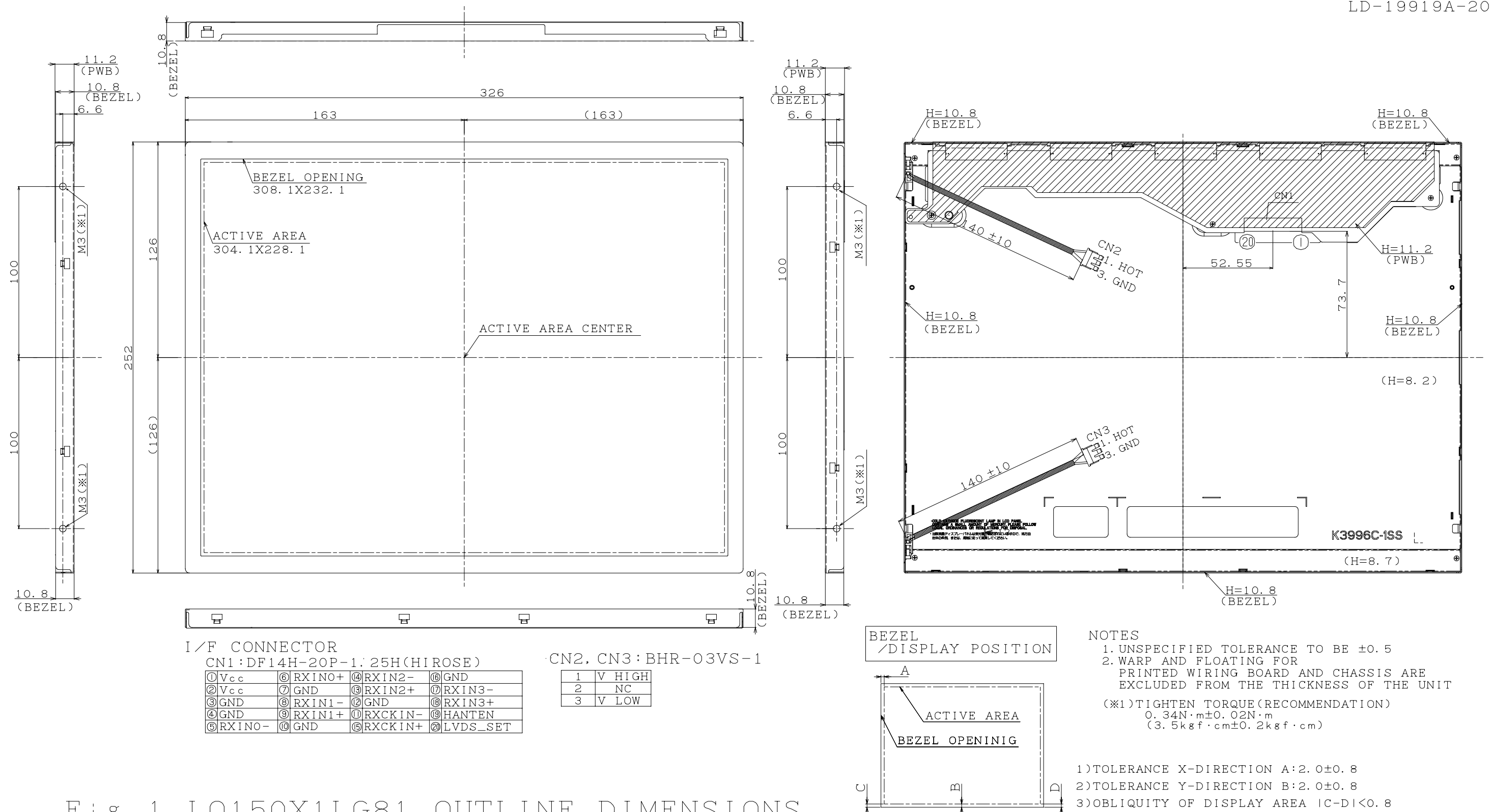
Fig. 1 LQ150X1LG81 OUTLINE DIMENSIONS
