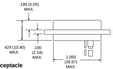
Receptacle
