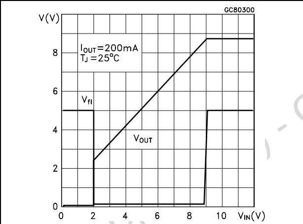
Figure 7. Output and flag voltage vs inp. volt.
