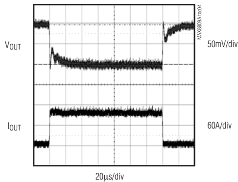
OUTPUT LOAD TRANSIENT
