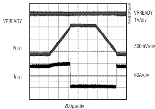
DYNAMIC VID RESPONSE
