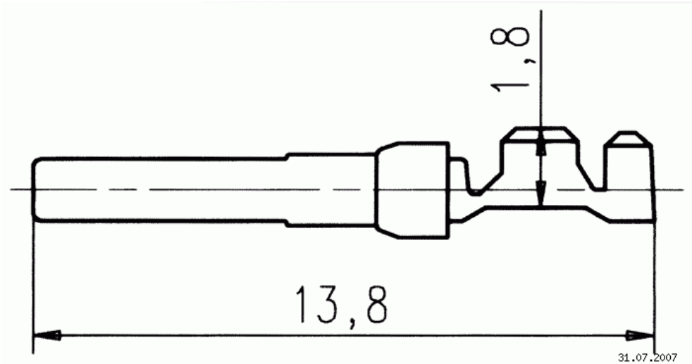
Ma zeichnung Dimensions in mm (Inch)
