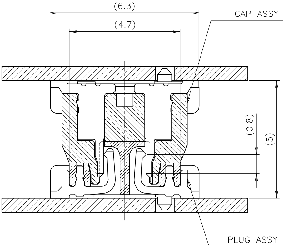
嵌合状態図
