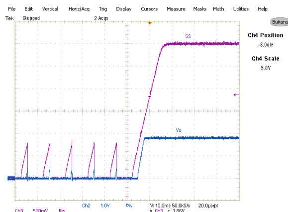
Fig. 12: Short (Hiccup) Recovery Ch 2 : V_{out} , Ch 3 : V_{ss}
