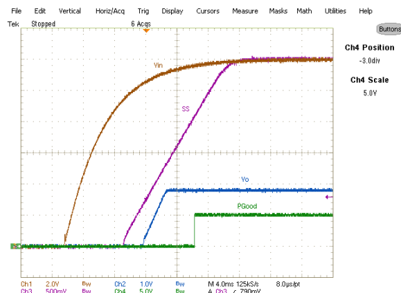
Fig. 8: Start up at 8A Load, Ch 1 : V_{in} , Ch 2 : V_{out} , Ch 3 : V_{ss} , Ch 4 : V_{PGood}
