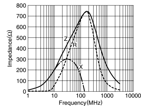
MPZ1608S601A
