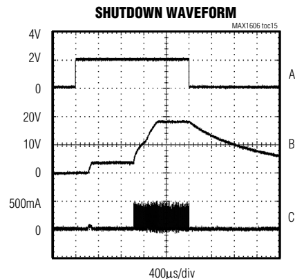
A: V_{SHDN} , 2V/div B: V_{OUT} , 10V/div , R_{OUT} = 1.8k\Omega C: I_{L1} , 500mA/div
