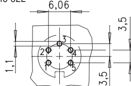
5 POL DIN 45 322
