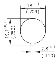
Montageausschnitt
