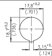
Montageausschnitt
