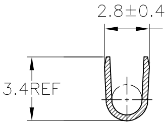
断面 A-A SECT A-A
