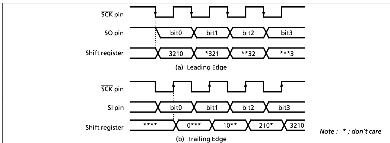
Figure 2-40. Shift Edge
