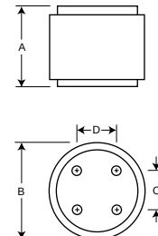
Fig. 3: 1500-2500 Amp Range
