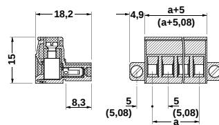
MSTB 2,5 HC/...-STF(-5,08)
