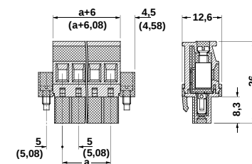
MVSTBW 2,5 HC/...-STF(-5,08)
