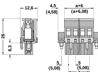
MVSTBR 2,5 HC/...-STF(-5,08)
