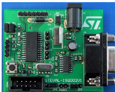
STEVAL-ISQ002V1
