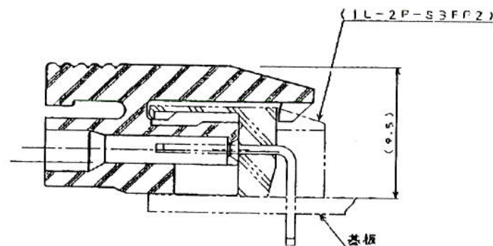
断面 A-A 及び組合せ状態図
