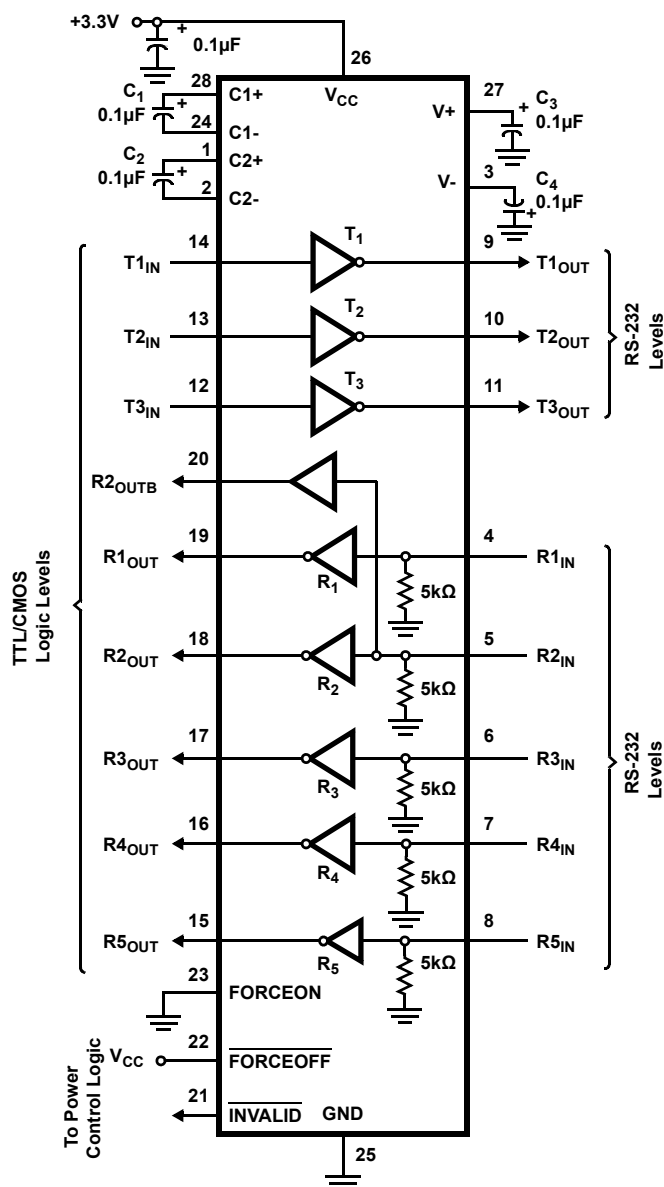
ICL3243
