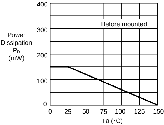
(3) SOT-23-5
