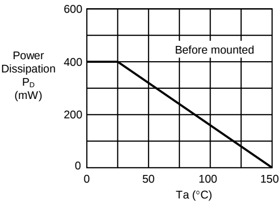
(1) TO-92
