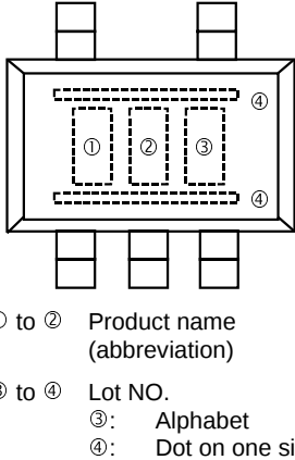
(3) SOT-23-5
