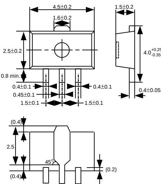
(2) SOT-89-3
