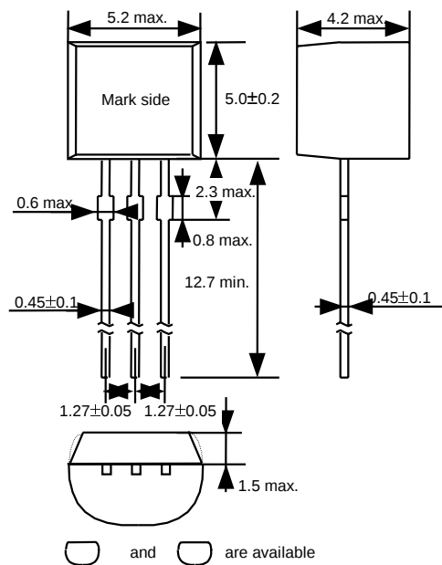
(1) TO-92
