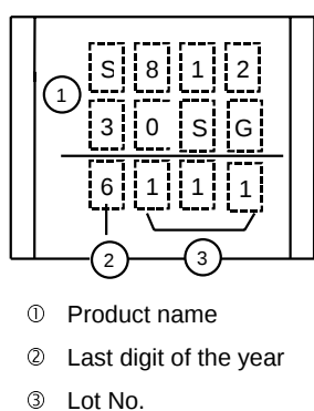
(1) TO-92
