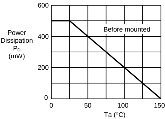
(2) SOT-89-3
