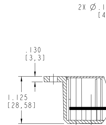
SECTION D-D
