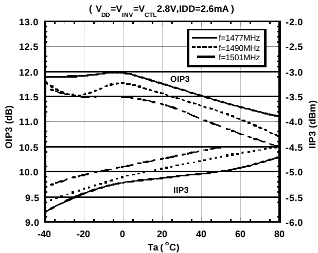
OIP3,IIP3 vs. Ta
