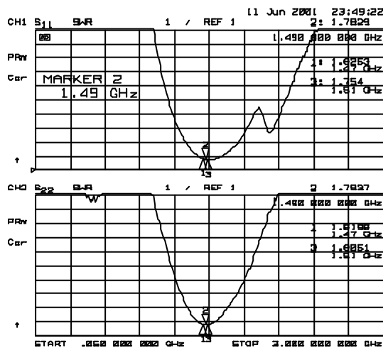
VSWR
