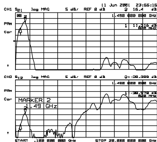
S21, S12
