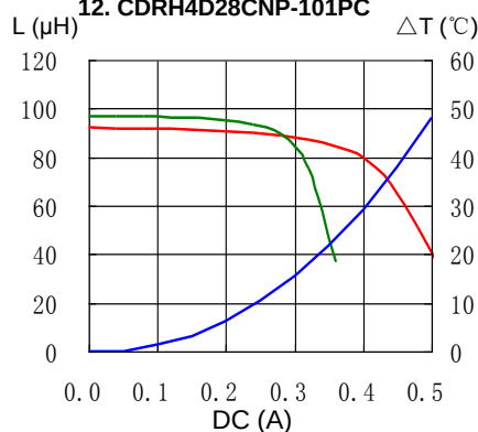
12. CDRH4D28CNP-101PC
