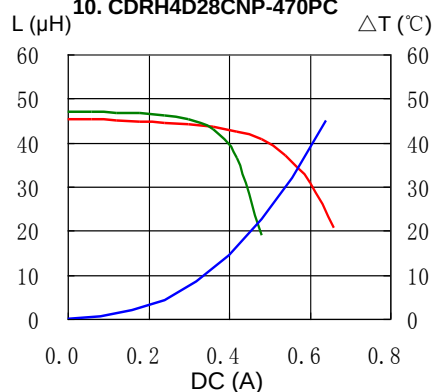
10. CDRH4D28CNP-470PC
