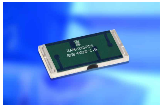
Bauform/Size 2512
