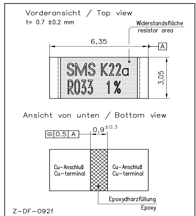
Bauform/Size 2512
