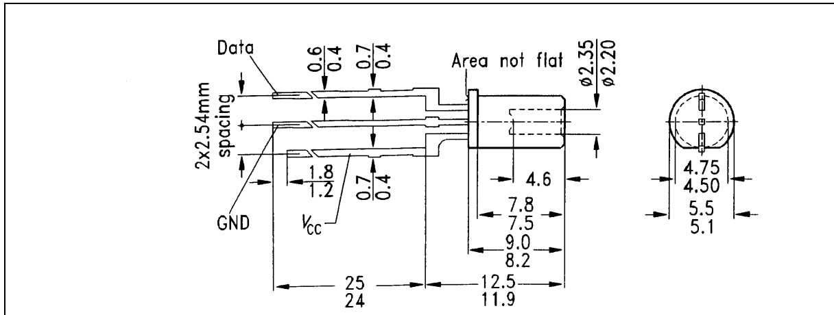
SFH 551/1
