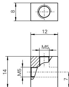
T-Stück (PT-300-M5)
