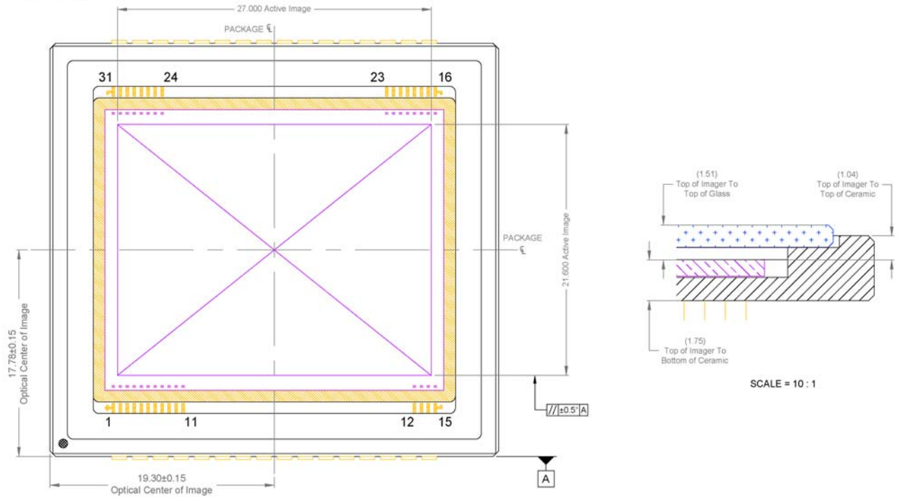
Figure 23. Die Placement
