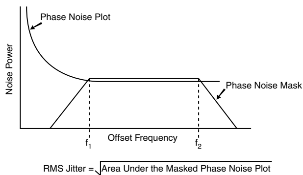
PHASE JITTER
