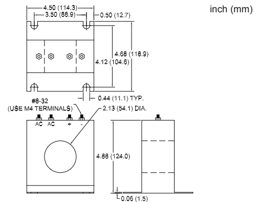
100-600 Aac input
