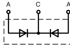
TO-3 P
