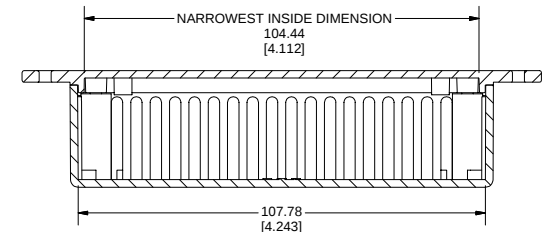
SECTION D-D
