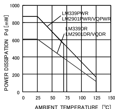
LM339DR/PWR LM2901DR/PWR/VQDR/VQPWR
