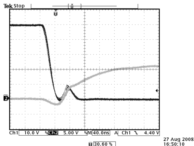
Figure 3. Q4 (CD Leg) at 15-A Load
