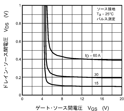
図 8.4 V_{DS} - V_{GS}
