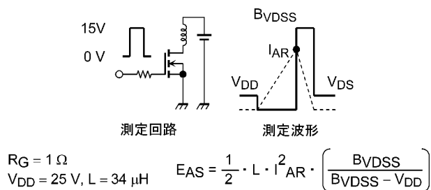
図 8.15 測定回路/測定波形
