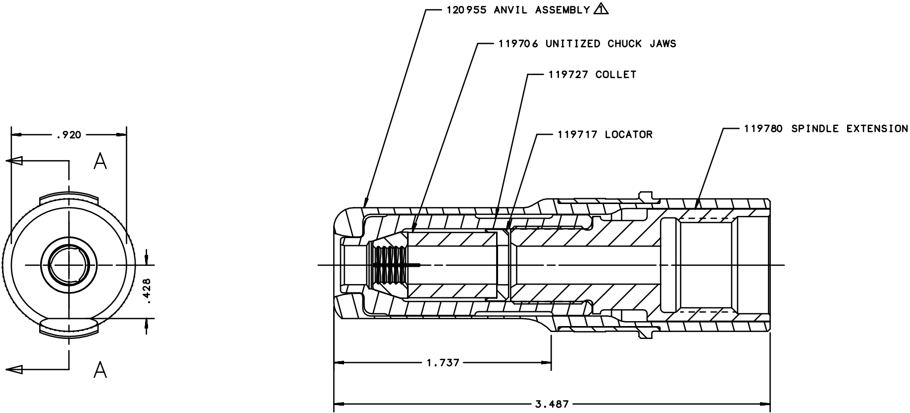
SECTION A-A
