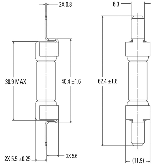
ZXPY Blade
