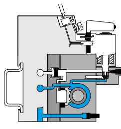
4/2 bistable module
