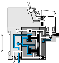
4/2 monostable module
