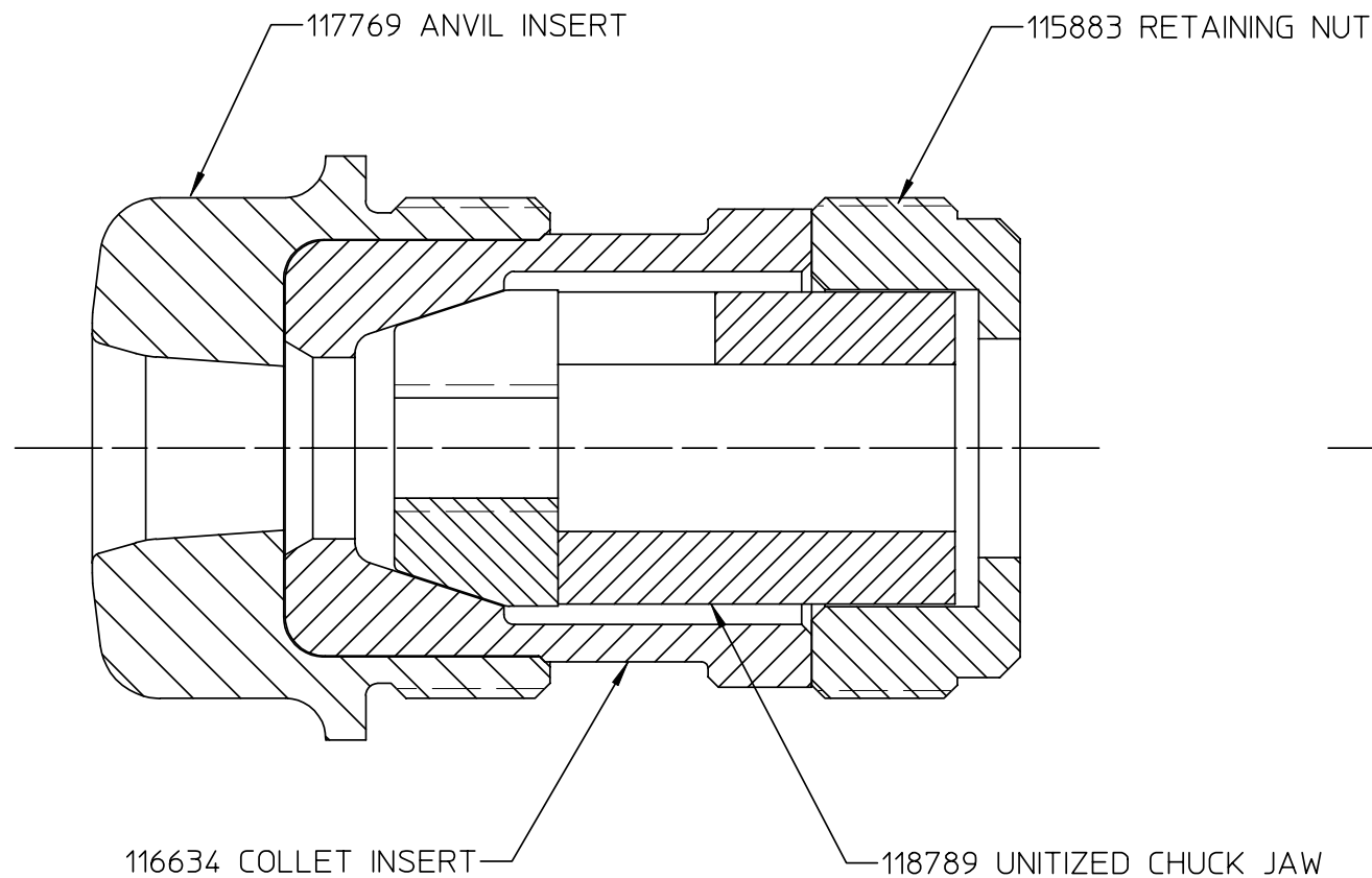
SECTION A-A
