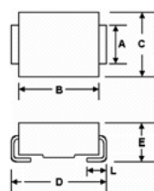
SMBJ (DO-214AA)
