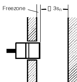
Fig.2: Shielded SUS type
