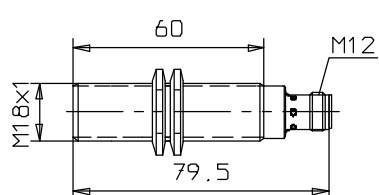
E2EL-X5□-M1L, E2EL-X8□-DM1L, E2EL-X8□-DM1SL
