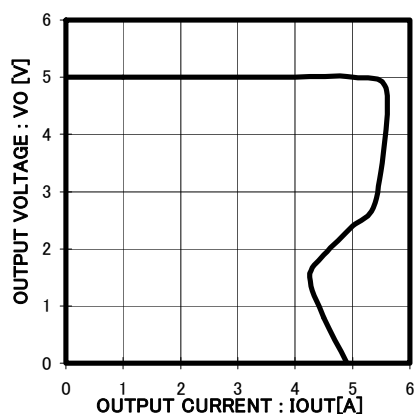
Fig.11 OCP VCC=20V
