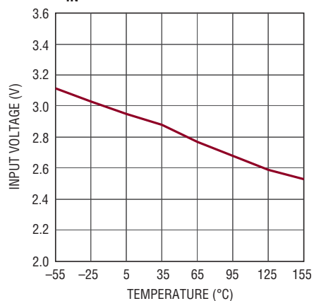
V_{IN} UVLO
