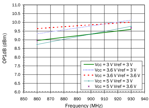
OP1dB
