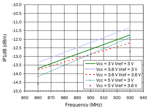
IP1dB
