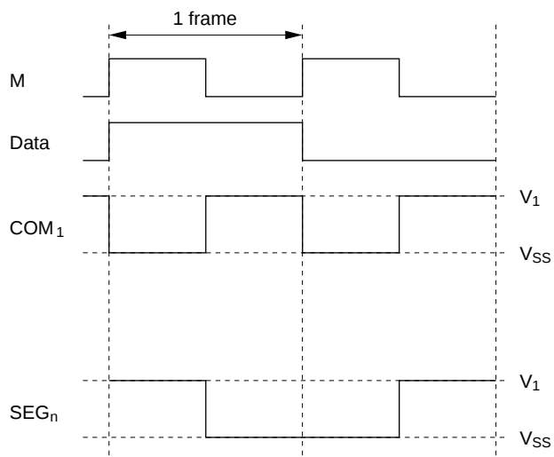
Figure 13-11 (d) Waveforms at Static Duty
